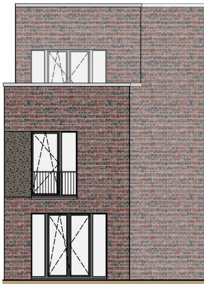
Ansicht Garten
